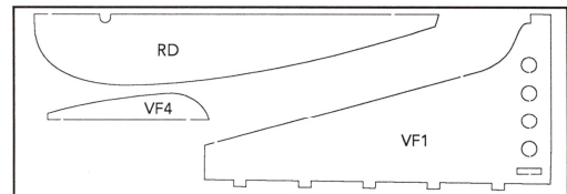
BP12 1/4" Balsa
